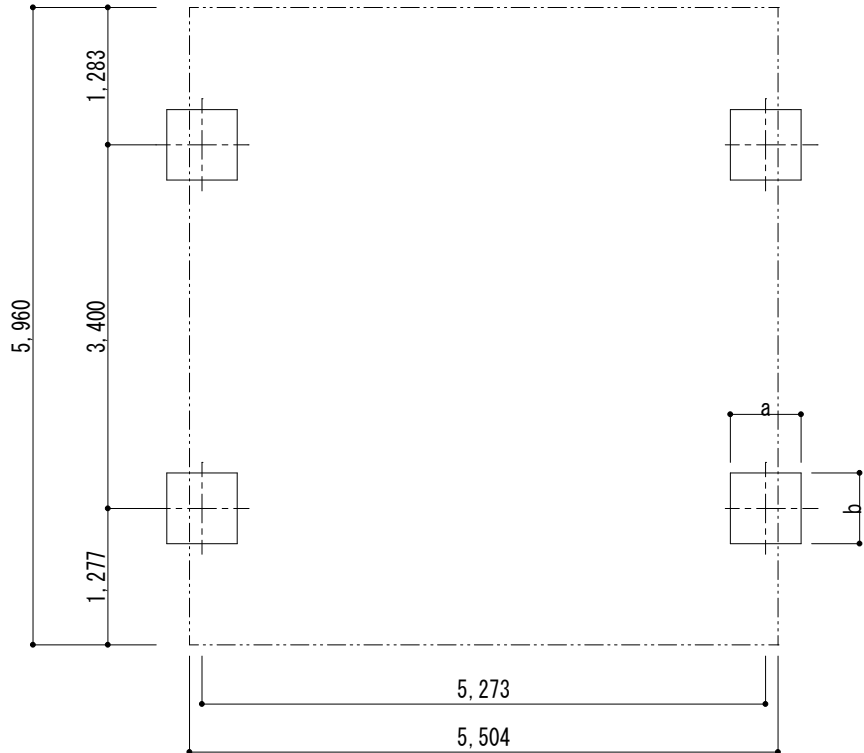
■ 基礎配置図
